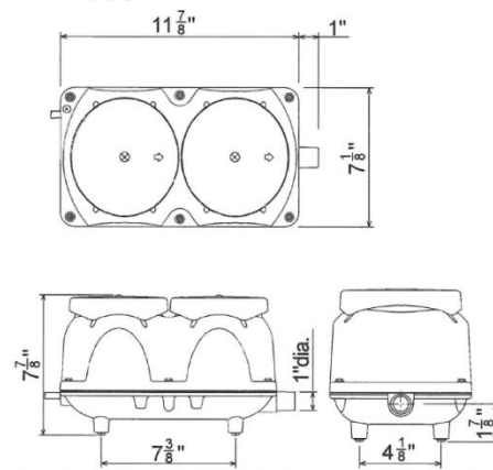
□MAC150RII/200RII
