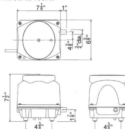
□MAC60RII/80RII/100RII
